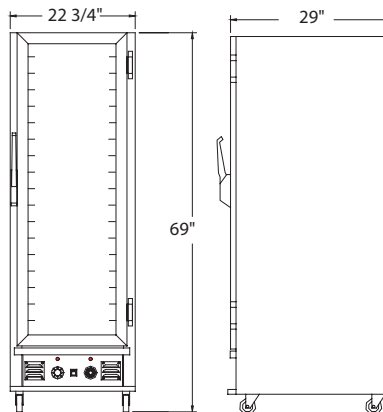
DP18 & DP18AD
